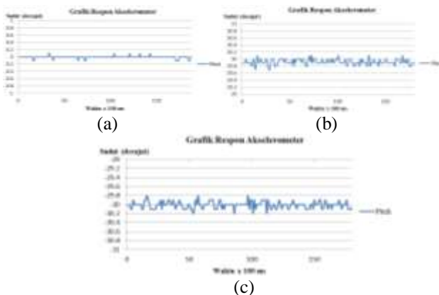
Gambar 7 respon akselero (a) sudut 0° (b) sudut 30° (c) sudut - 30°
