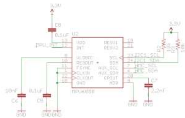
Gambar 2. Rangkaian MPU6050
