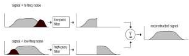
Gambar 3. Prinsip kerja tapis komplementer [5].
