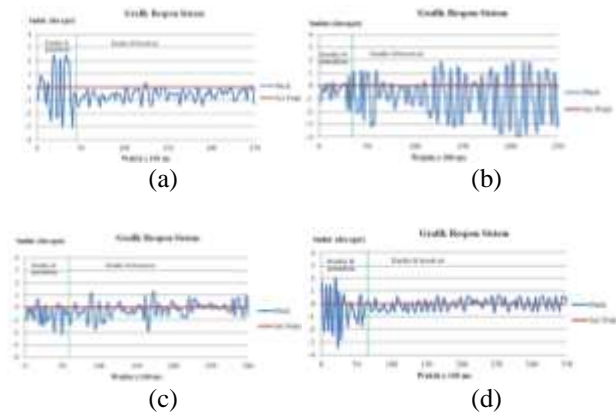
Gambar 11 Respon Remotely Operated Vehicles (ROV) dengan nilai parameter (a) K_p=15 , K_i=0 , dan K_d=0 (b) K_p=20 , K_i=0 , dan K_d=0 (c) K_p=15 , K_i=0,01 , dan K_d=1 (d) K_p=15 , K_i=0,01 , dan K_d=5
