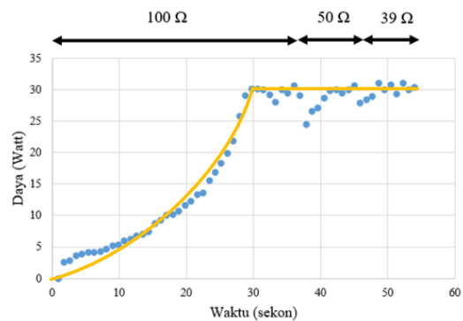
Gambar 13. Grafik MPPT iradiasi 1092 W/m 2 dan suhu 29°C
