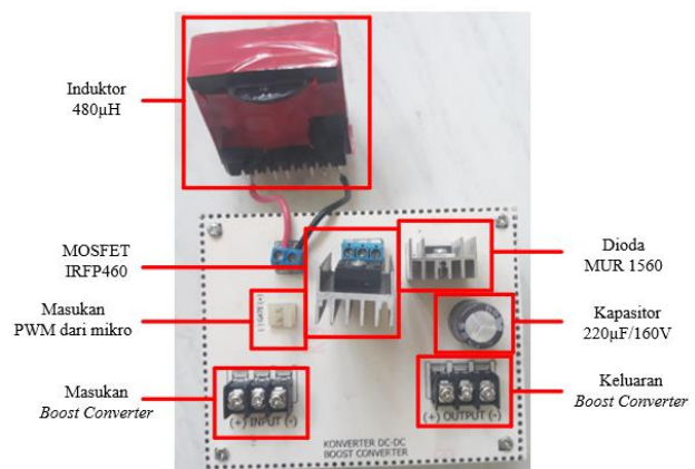
Gambar 1. Realisasi rangkaian boost converter
