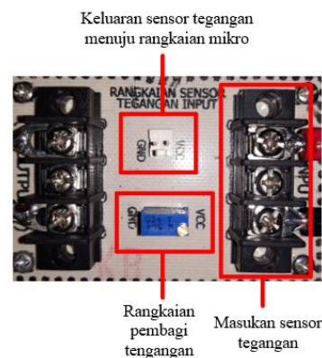
Gambar 3. Realisasi sensor tegangan
