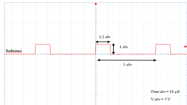
Gambar 11. Gelombang keluaran PWM duty cycle 25%
