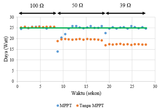
Gambar 16. Grafik perbandingan sistem MPPT dan tanpa MPPT iradiasi 752 W/m 2 dan suhu 29°C
