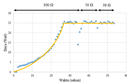
Gambar 14. Grafik MPPT iradiasi 752 W/m 2 dan suhu 29°C
