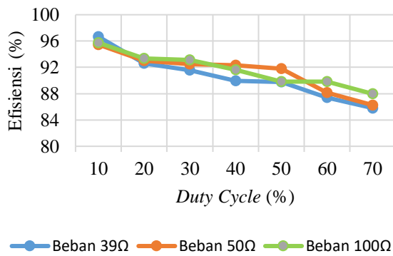
Gambar 10. Efisiensi boost converter variasi duty cycle
