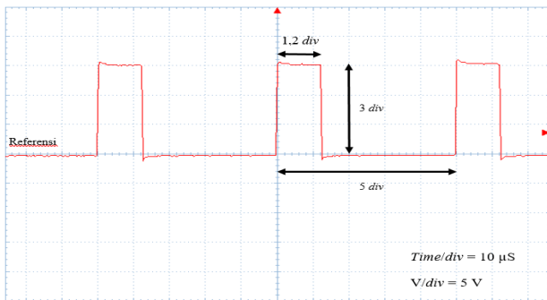
Gambar 12. Gelombang keluaran PWM TLP250 duty cycle 25%
