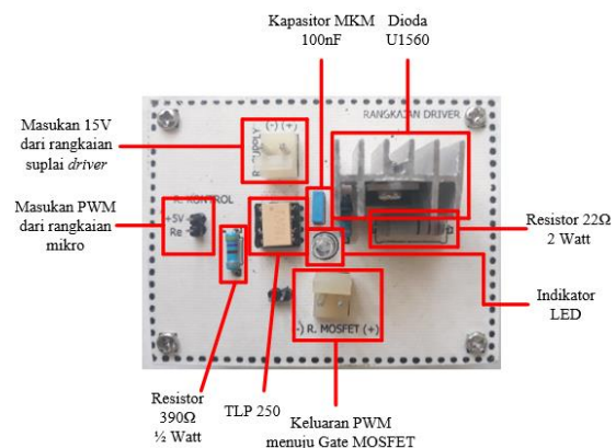
Gambar 4. Realisasi rangkaian driver MOSFET
