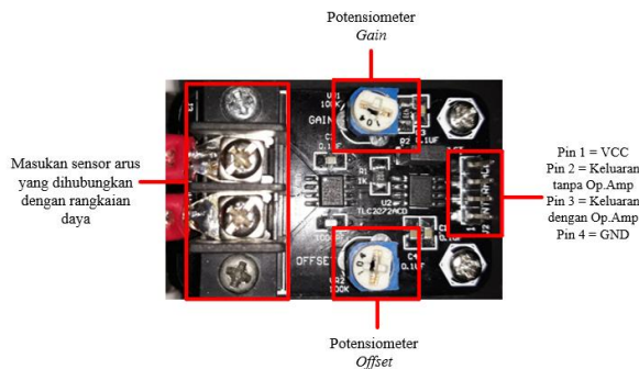
Gambar 2. Realisasi sensor arus
