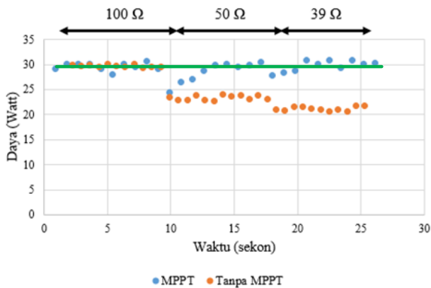
Gambar 15. Grafik perbandingan sistem MPPT dan tanpa MPPT iradiasi 1092 W/m 2 dan suhu 29°C
