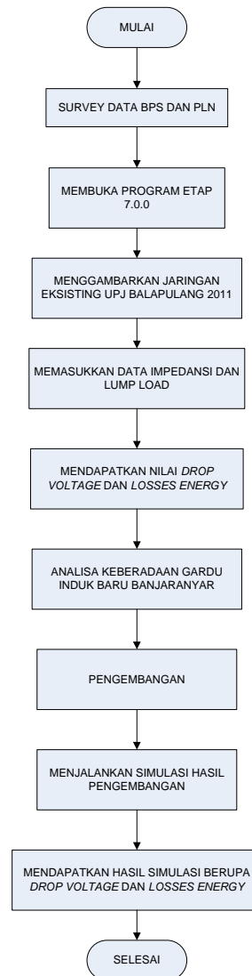
Gambar 5. Diagram Alir Simulasi ETAP 7.0.0
