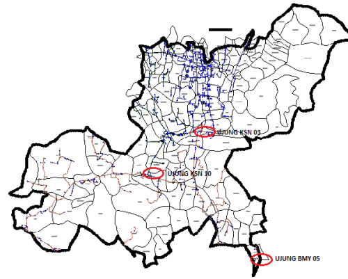
Gambar 8. Ujung feeder BMY 05, KSN 03 dan KSN 10 yang tidak memenuhi kriteria dari PT. PLN
