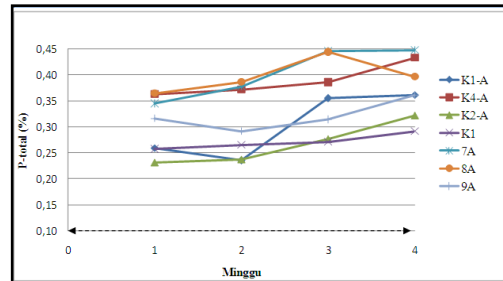
Gambar 19 : Grafik Perubahan P-Total Aktivator Lumpur Aktif
