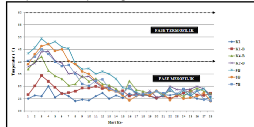
Gambar 2 : Grafik Perubahan Temperatur Aktivator EM4
