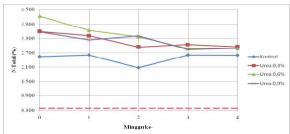
Gambar 12. Grafik Perubahan N-Total Pada Pengomposan Sampah Sayuran
