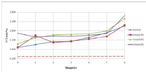
Gambar 13. Grafik Perubahan N-Total Pada Pengomposan Sampah Campuran
