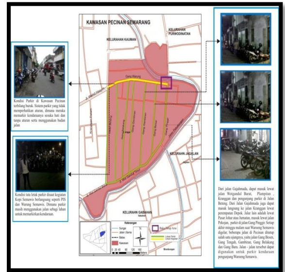
Gambar 3 Kondisi Parkir
