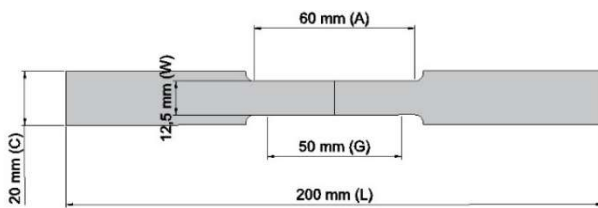
Gambar 3. Dimensi Spesimen Uji Tarik [22]
