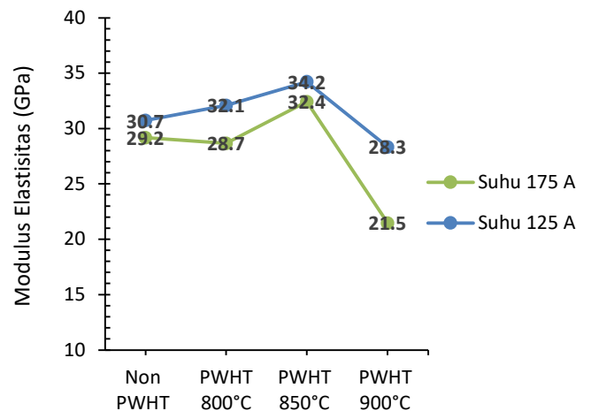
Gambar 8. Nilai Modulus Elastisitas (GPa)
