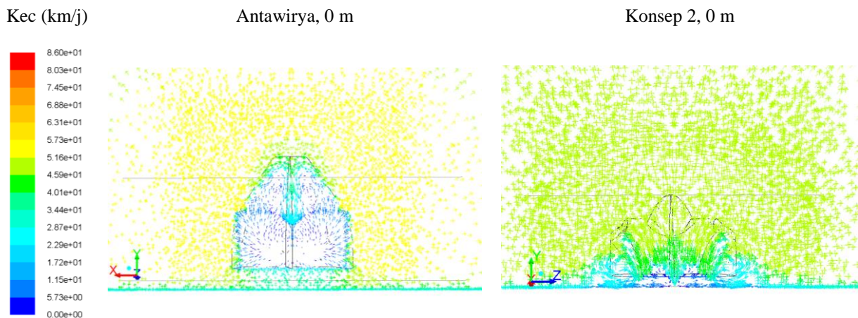
Gambar 11. Vektor kecepatan bidang vertikal pada 50 km/j.
