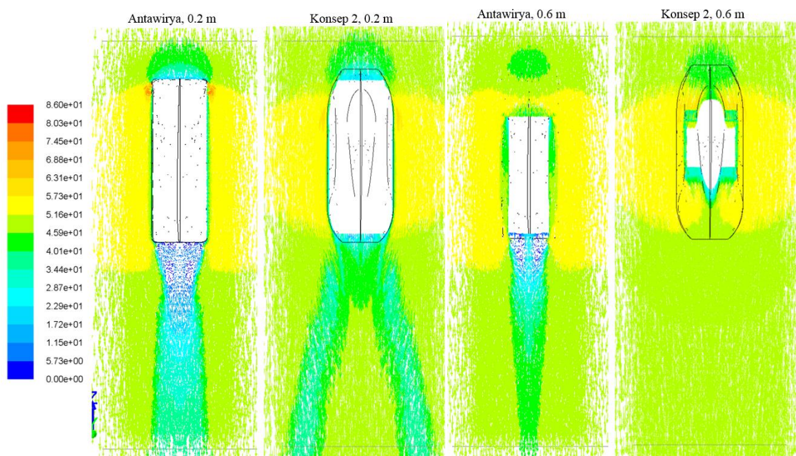
Gambar 10. Vektor kecepatan bidang horizontal pada 50 km/j.
