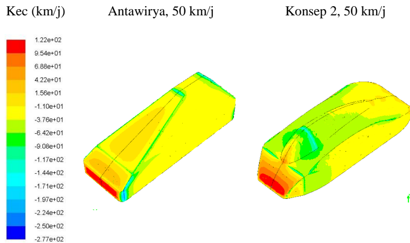
Gambar 13. Kontur tekanan statis tampak isometric pada 50 km/j.
