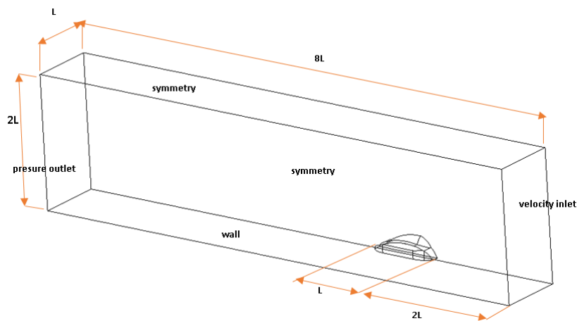
Gambar 6. Geometri Konsep 2 dan wind tunnel dengan ANSYS Design Modeller .
