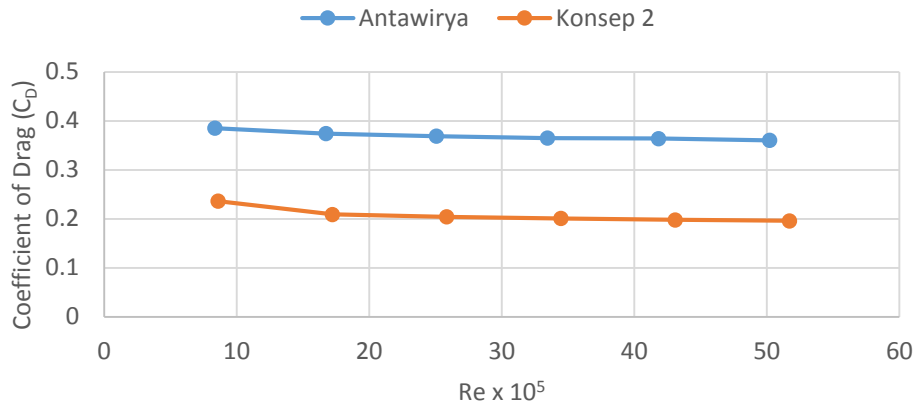
Gambar 9. Grafik perbandingan C D Antawirya vs C D Konsep 2 terhadap bilangan Reynold.
