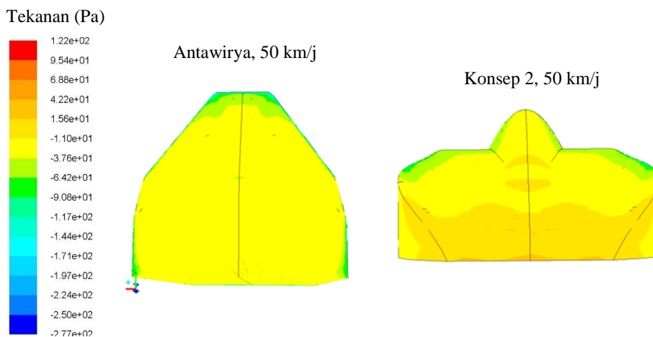
Gambar 14. Kontur tekanan statis tampak belakang pada 50 km/j.
