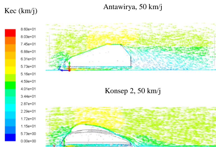
Gambar 12. Vektor kecepatan bidang simetri pada 50 km/j.
