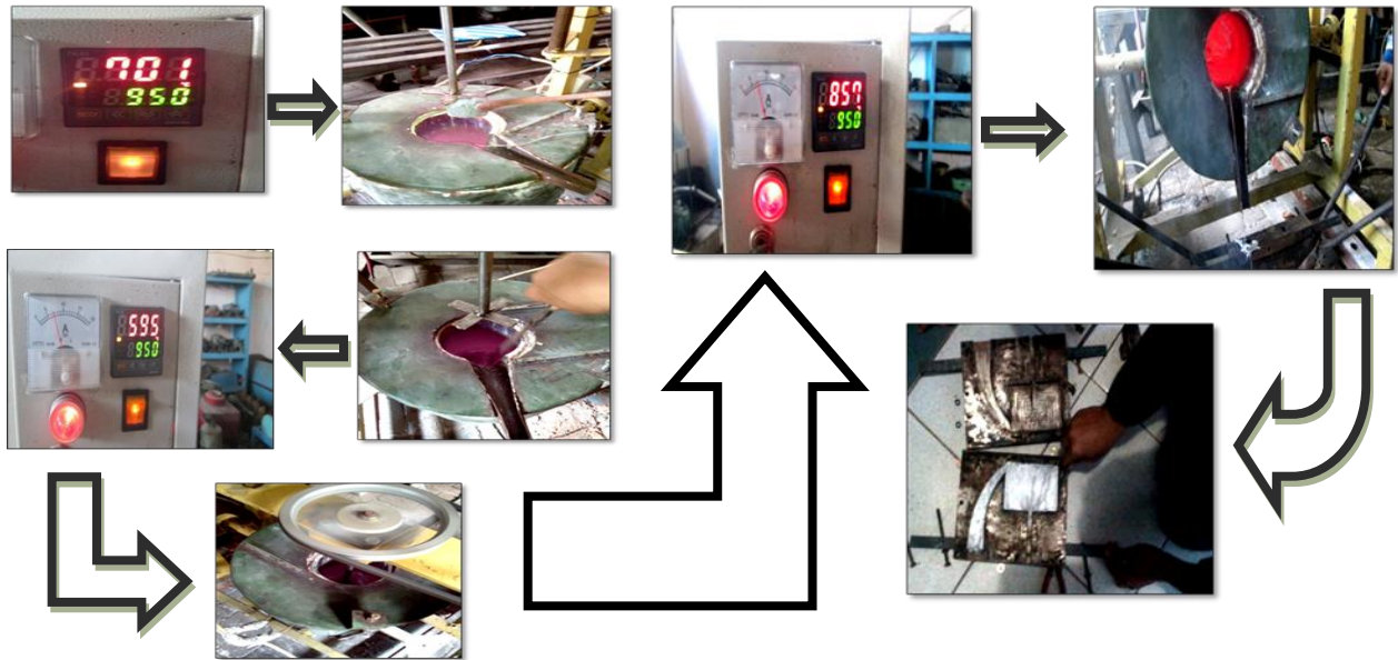
Gambar 3. Proses pengadukan dan penuangan AlSiC.
