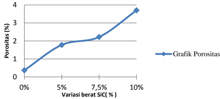
Gambar 4. Grafik hubungan nilai porositas rata-rata pada komposit Al-SiC
