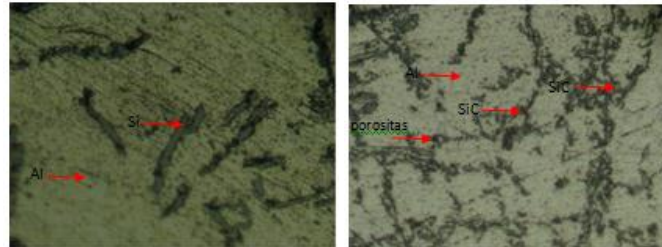
Gambar 7. (a) Struktur mikro komposit Al-SiC dengan SiC 0% (b) Struktur mikro komposit Al-SiC dengan SiC 5%
