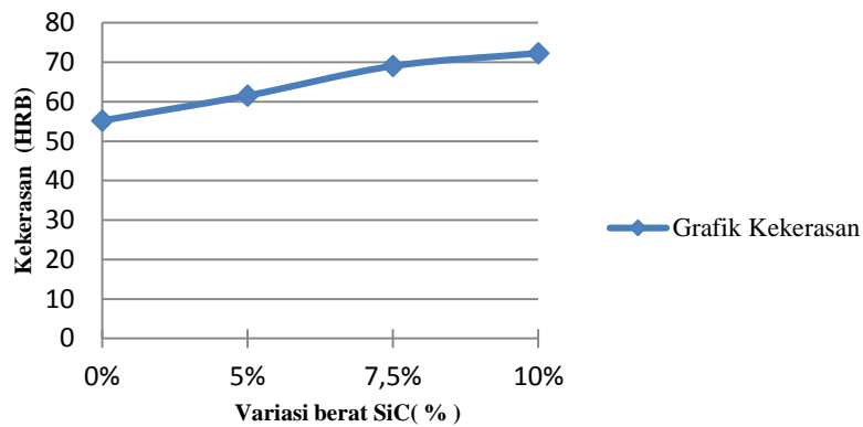
Gambar 5. Grafik perbandingan nilai kekerasan rata-rata pada komposit Al-SiC dengan variasi berat SiC
