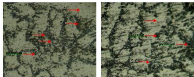
Gambar 8. (a) Struktur mikro komposit Al-SiC dengan SiC 7,5% , (b) Struktur mikro komposit Al-SiC dengan SiC 10%
