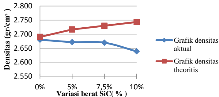
Gambar 3. Grafik nilai densitas rata-rata pada komposit AlSi-SiC dengan variasi berat SiC
