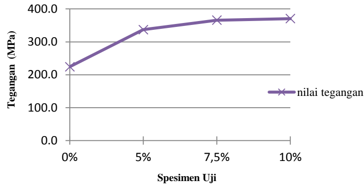
Gambar 6. Grafik perbandingan tegangan maksimum rata-rata pada komposit Al-SiC dengan variasi berat SiC
