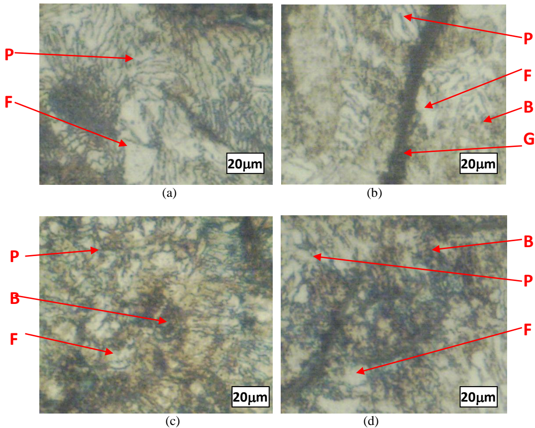
Gambar 14. Evolusi struktur mikro besi cor kelabu jenis FC 30
