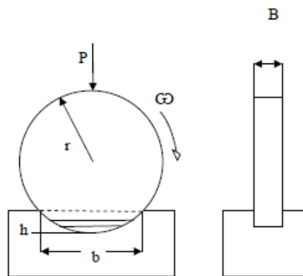
Gambar 7. Skema Ilustrasi pengujian Aus Ogoshi
