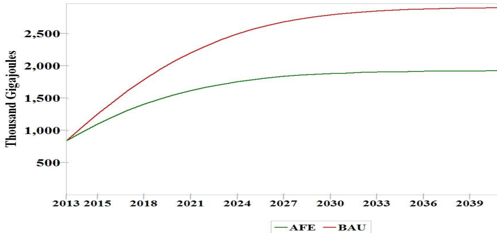
Gambar 2. Grafik Kebutuhan energi dengan metode business as usual dan metode advanced fuel economy hingga tahun 2040
