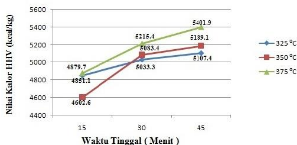
Gambar 7. Grafik Hasil Nilai Kalor Biobriket Komposisi 50% Kulit Mete – 50% Sekam Padi.
