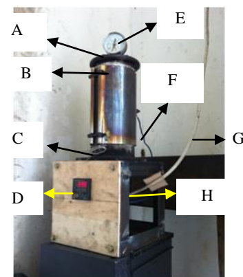
Gambar 6. Instalasi Alat - Alat Uji Pirolisa.
