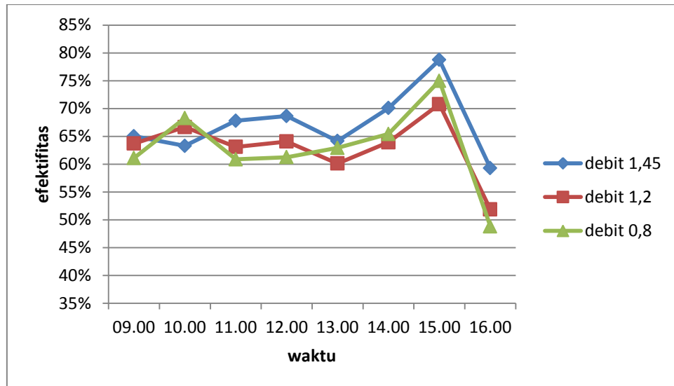
Gambar 8. Grafik efektifitas evaporative cooling tanggal 4 November 2013
