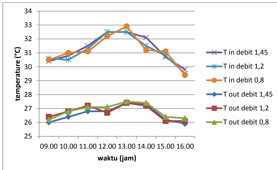
Gambar 3. Grafik T in vs T out tanggal 1 November 2013
