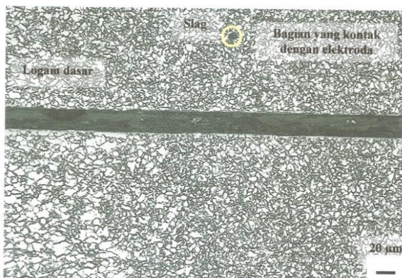
Gambar 3. Hasil pengamatan mikrofografi (perbesaran 20 µm) untuk nugget las titik SIR dengan arus 8.6 A dan waktu pengelasan selama 10 detik.
