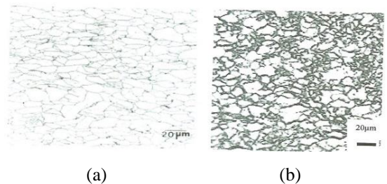
Gambar 6. (a) Struktur mikro UNS G10080 steel di normalisasi pada 20 µm daerah gelap adalah pearlite dan daerah terang adalah ferrit . (b) Struktur mikro logam dasar yang digunakan pada pengelasan titik baik dengan mesin las titik SIR maupun las titik acuan pada perbesaran 20µm, yaitu AISI 1010. Daerah terang adalah ferit dan daerah gelap adalah perit.
