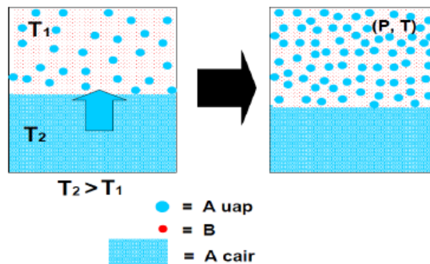
Gambar 2. Skema proses humidifikasi
