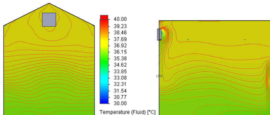
Gambar 11. Kontur suhu pada centre plane (Atas: Tampak samping , bawah: tampak depan )
