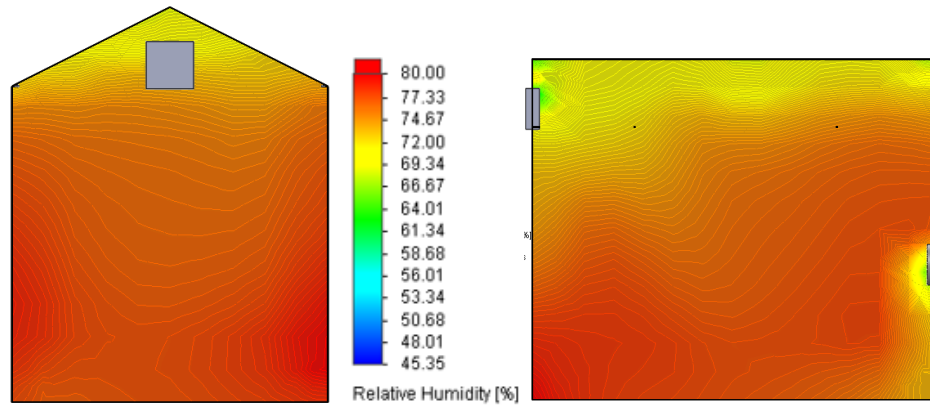
Gambar 10. Kontur RH pada centre plane (Atas: Tampak samping , bawah: tampak depan )
