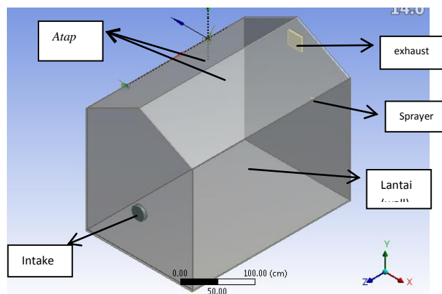
Gambar 6. Kondisi batas yang diterapkan pada domain komputasi.
