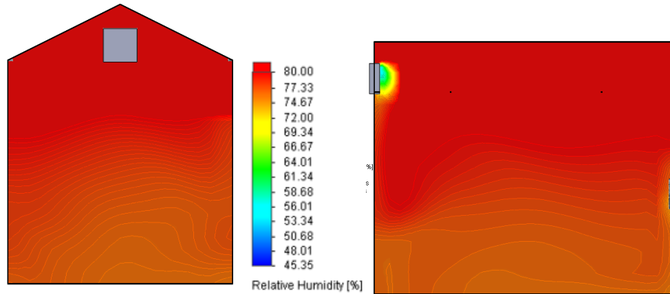
Gambar 12. Kontur RH pada centre plane (Atas: Tampak samping, bawah: tampak depan)
