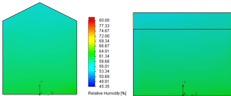
Gambar 8. Kontur RH pada Kasus 1
