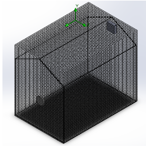
Gambar 5. Penggenerasian mesh
