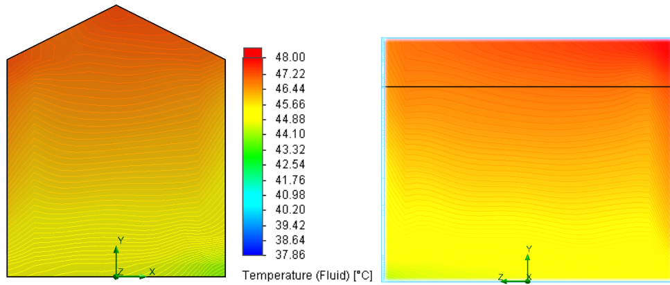
Gambar 7. Kontur suhu pada Kasus 1
