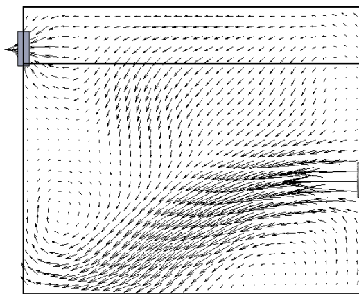
Gambar 13. Velocity vector pada center plane tampak samping
