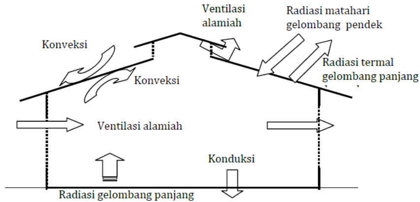
Gambar 1. Proses perpindahan panas pada empat subsistem Rumah Tanaman [3]
