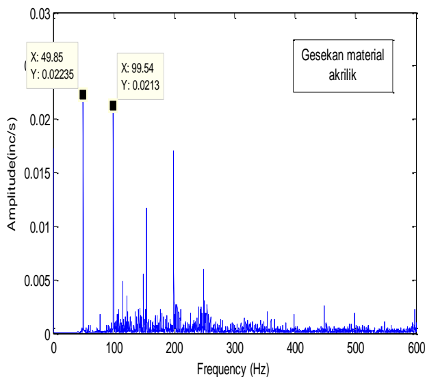
Gambar 17. Akrilik rub (3000 rpm)
