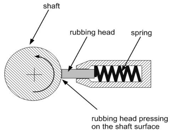
Gambar 3. Ujung rubbing menekan melawan poros [5].
