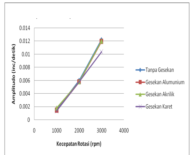
Gambar 12. Maksimum kedua (vertikal)
