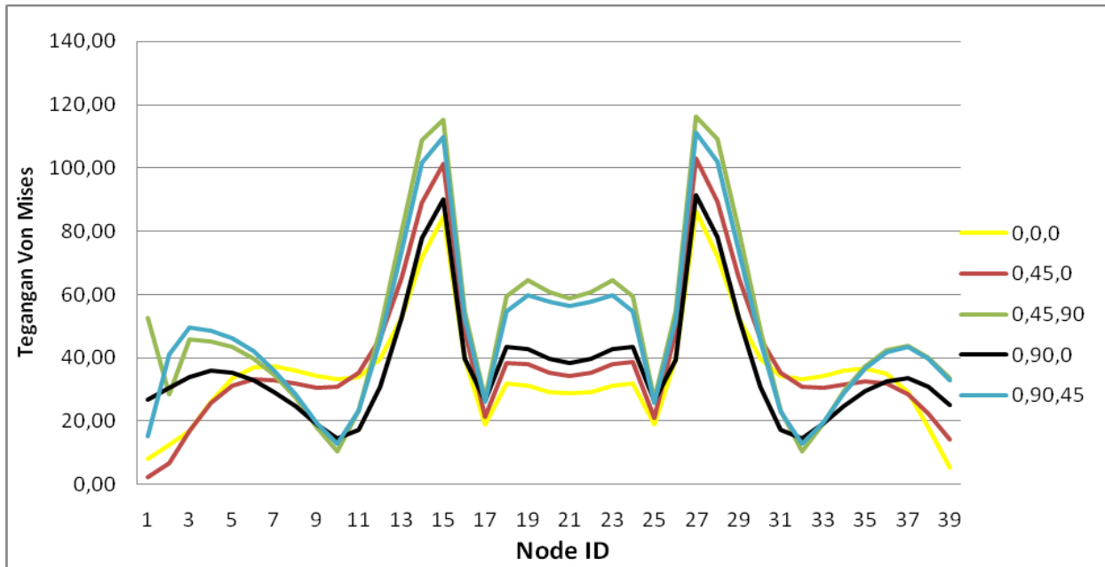
Gambar 6. Distribusi tegangan Von Mises setiap material
