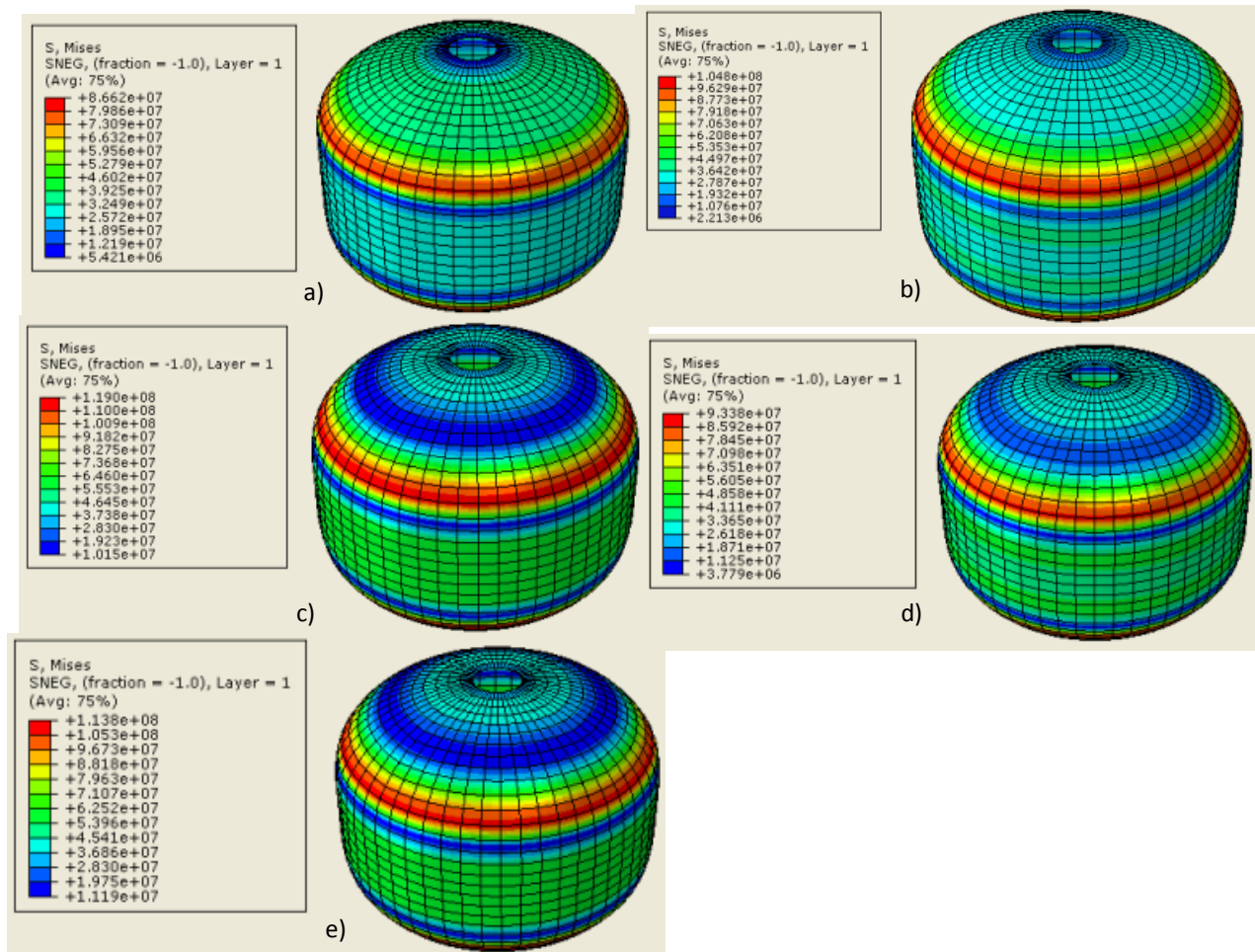
Gambar 5. Distribusi tegangan von mises pada struktur tabung gas perlakuan pembebanan statis material GFRP : (a)UD, (b)0,45,0, (c)0,90,0, (d)0,45,90, (e)0,90,45
