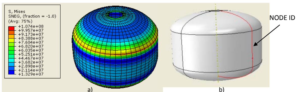
Gambar 3. LPG 3kg material SG295: a) distribusi tegangan von misses , b) Letak node untuk distribusi tegangan,
