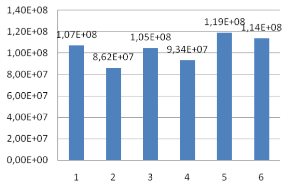
Gambar 7. Grafik Perbandingan tegangan Von Mises
