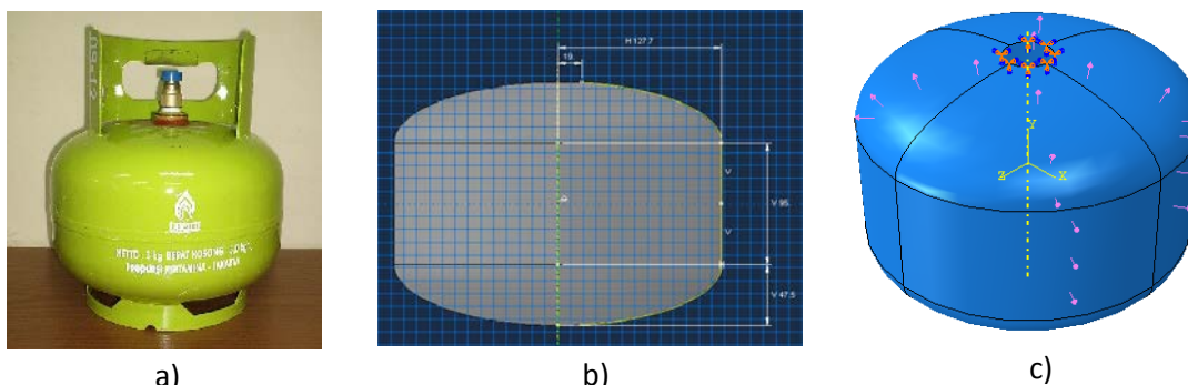
Gambar 2. Tabung LPG 3 kg: a) (SNI 1452:2007), b) parameter geometri, c) kondisi batas dan load
