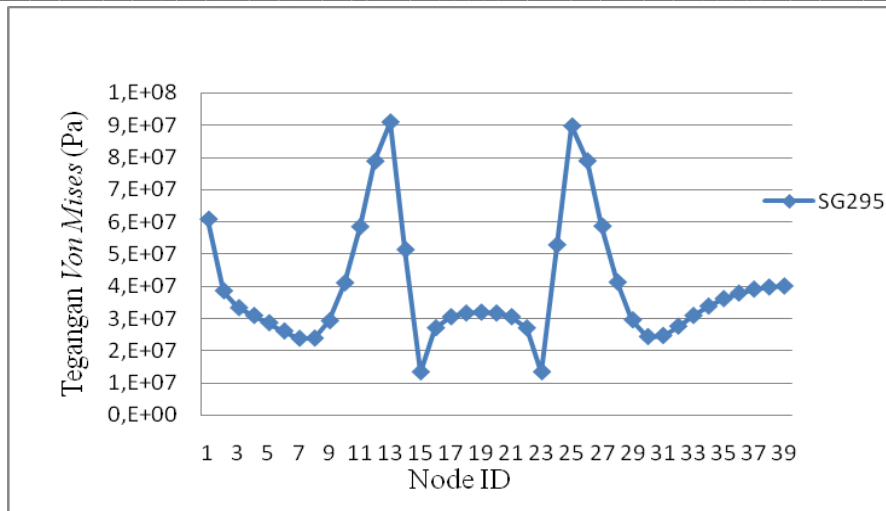
Gambar 4. Grafik distribusi tegangan SG295
