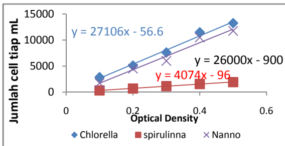
Gambar 2. Grafik OD vs Biomassa
