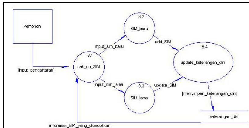
Gambar 7 DFD Level 2 Proses Add_keterangan_diri
