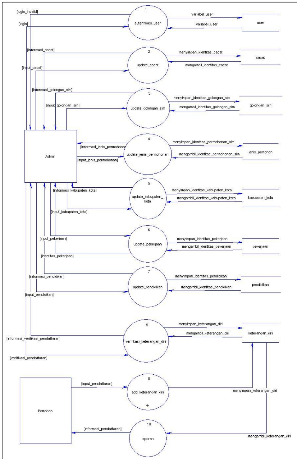
Gambar 6 DFD Level 1
