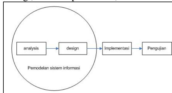
Gambar 2 Sekuensial Linear
