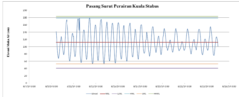
Gambar 2. Fluktuasi pasang surut, Pelabuhan Kuala Stabas, Krui, Lampung Barat (sumber: pengolahan data pengamatan, 2015)
