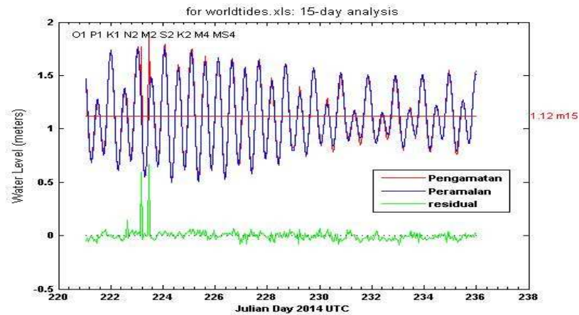
Gambar 3. Grafik verifikasi elevasi muka air lapangan dengan modelWORLD TIDES (sumber: pengolahan data pengamatan, 2015)
