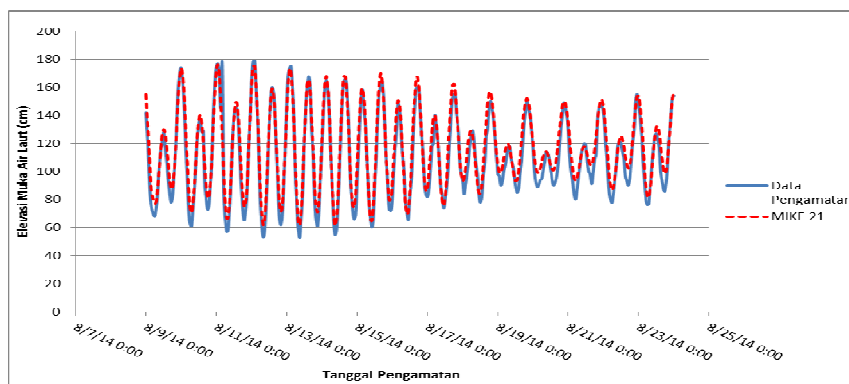
Gambar 5. Grafik verifikasi elevasi muka air lapangan dengan model MIKE 21 (sumber: pengolahan data pengamatan, 2015)
