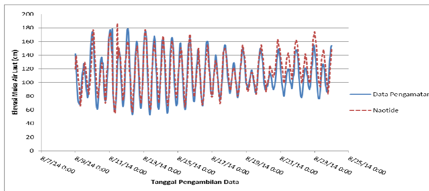
Gambar 4. Grafik verifikasi elevasi muka air lapangan dengan model NAO Tide (sumber: pengolahan data pengamatan, 2015)
