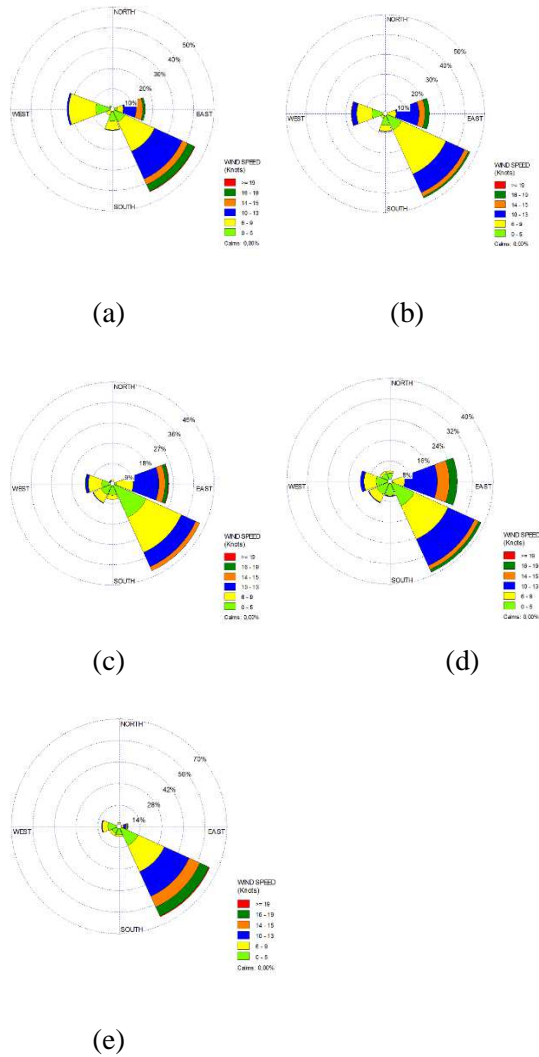
Gambar 1. Mawar Angin (a)Tahun 2005, (b)Tahun 2006, (c) Tahun 2007, (d)Tahun 2008, (e) Tahun 2009
