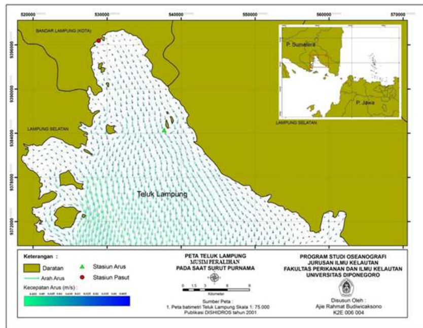
Gambar 14. Pola Arus Saat Surut Terendah Purnama pada Musim Peralihan Perairan Teluk Lampung.
