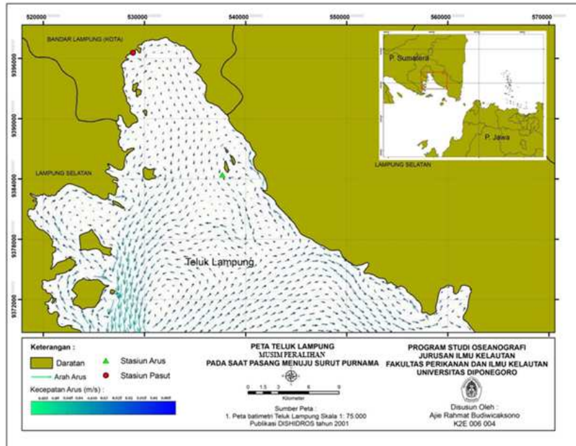
Gambar 13. Pola Arus Saat Pasang Tertinggi Menuju Surut Terendah Purnama pada Musim Peralihan Perairan Teluk Lampung.
