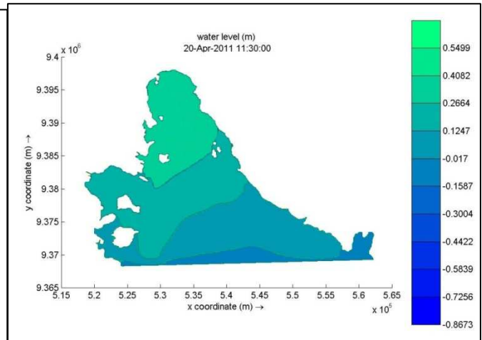
Gambar 3. Sebaran mendatar elevasi muka air pada saat muka air di titik pengamatan pasut berada saat muka air tertingggi menuju muka air terendah pada simulasi di Perairan Teluk Lampung.
