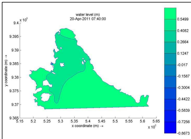
Gambar 2. Sebaran mendatar elevasi muka air pada saat muka air di titik pengamatan pasut berada saat muka air laut tertinggi pada simulasi di Perairan Teluk Lampung.
