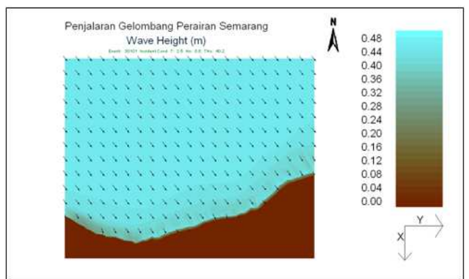
Gambar 6. Penjalaran gelombang dengan sudut datang gelombang dalam skenario model 22,8^{\circ} (Musim Timur)
