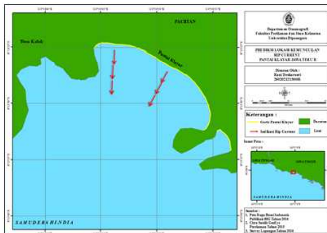
Gambar 5. Prediksi Lokasi Kemunculan Rip Current Pantai Klayar Jawa Timur.
