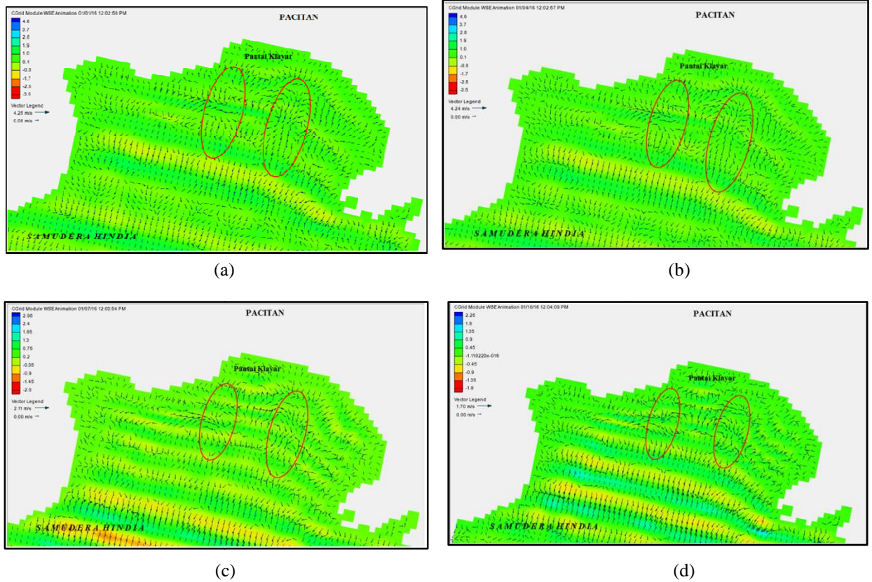
Gambar 4. Simulasi Model Rip Current (a) Musim Barat (b) Musim Peralihan I (c) Musim Timur (d) Musim Peralihan II
