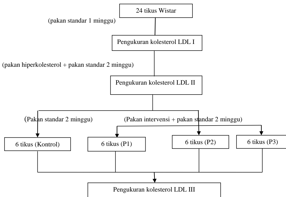
Gambar 1. Rancangan Penelitian
