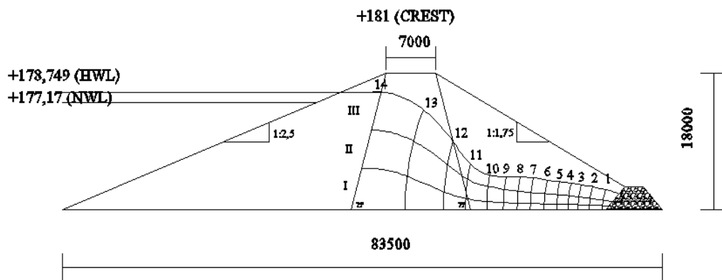
Gambar 6. Jaringan Trayektor Aliran Filtrasi
