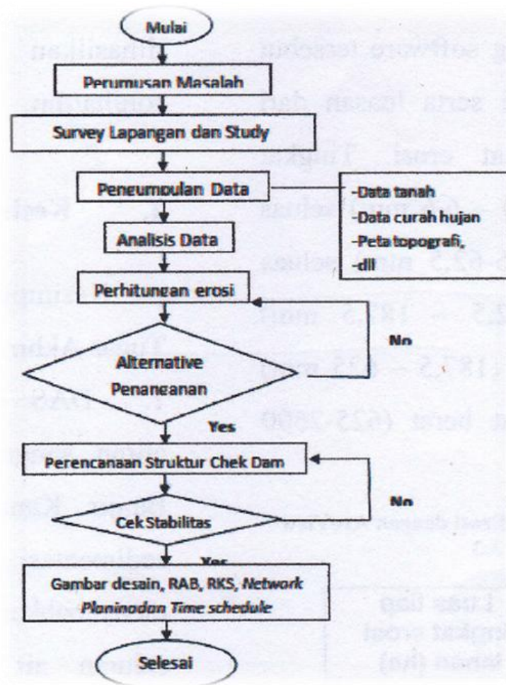
Gambar 3. Diagram alir perencanaan Check Dam
