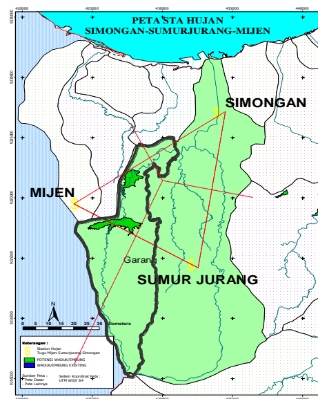
Gambar 1. Luas DAS Pengaruh 3 Stasiun Curah Hujan Sungai Kreo
