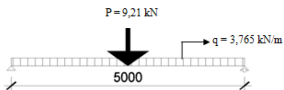
Gambar 4. Pemodelan pembebanan plat lantai
