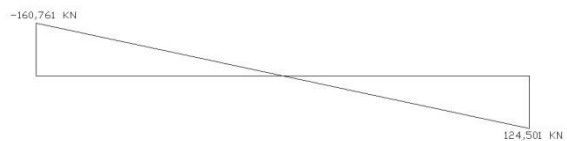
Gambar 2. Diagram Gaya Lintang pada Balok
