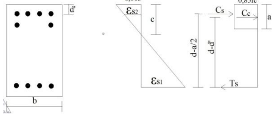
Gambar 4. Diagram Regangan dan Gaya Dalam Kondisi 2
