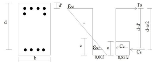
Gambar 3. Diagram Regangan dan Gaya Dalam Kondisi 1
