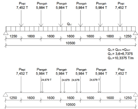
Gambar 5. Variasi model pembebanan pada balok melintang ( cross girder ).
