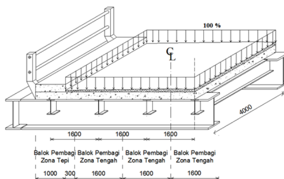
Gambar 2. Skema pembebanan BTR pada permukaan perkerasan jembatan.
