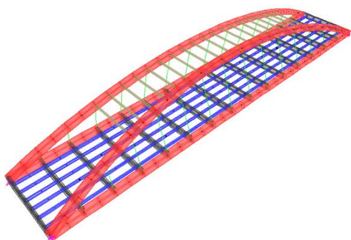
Gambar 6. Pemodelan Struktur Utama dengan program SAP2000
