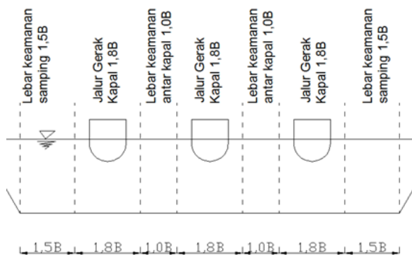
Gambar 1. Rencana alur pelayaran
