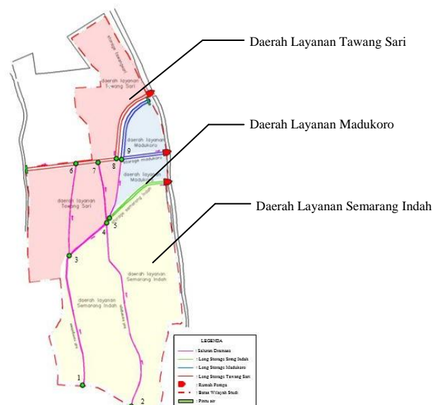
Gambar 2. Perencanaan Sistem Drainase Tawang Sari dan Tawang Mas
