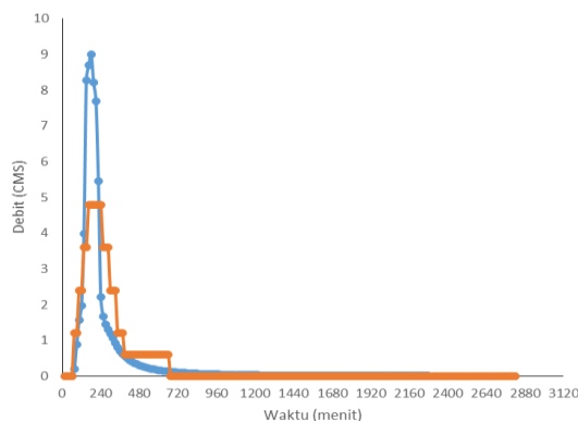
Gambar 8. Hidrograf Inflow dan Outflow Long Storage Madukoro
