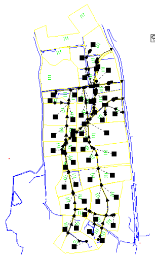
Gambar 3. Pemodelan Sistem Drainase Tawang Sari dan Tawang Mas
