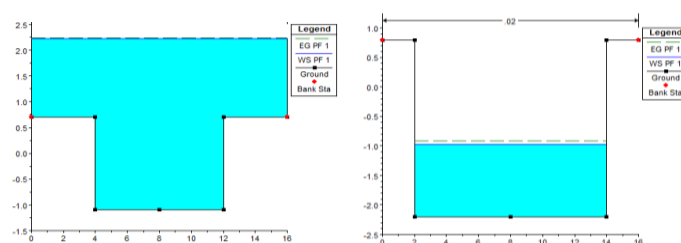
Gambar 6. Hasil Pemodelan HEC-RAS pada Long Storage Tawang Sari
