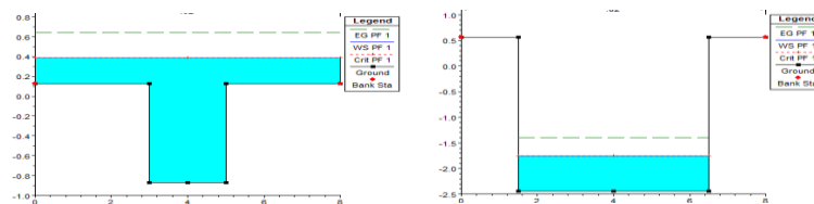
Gambar 5. Hasil Pemodelan HEC-RAS pada Long Storage Madukoro
