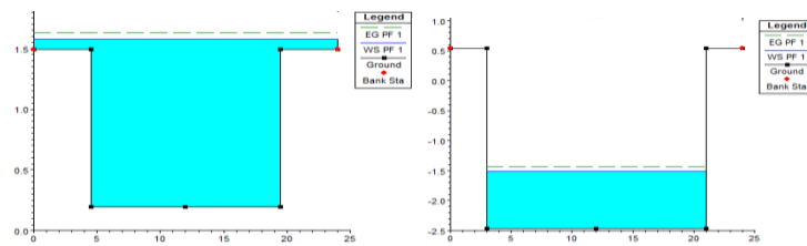
Gambar 4. Hasil Pemodelan HEC-RAS pada Long Storage Semarang Indah
