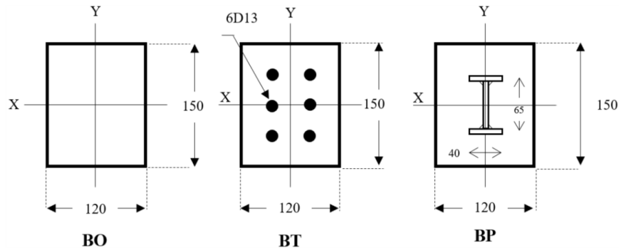
Gambar 1. Penampang Benda Uji
