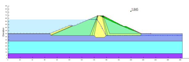
b. Slope/W sf 1,94
