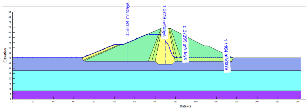
Gambar 5. Pemodelan stabilitas lereng kondisi steady state
