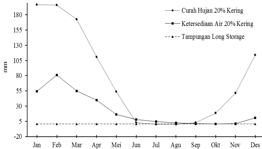
Gambar 7. Curah Hujan, Ketersediaan Air, dan Tampungungan Long Storage
