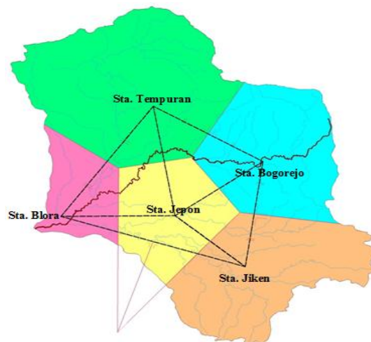
Gambar 3. Luas Pengaruh Tiap Stasiun Metode Poligon Thiessen
