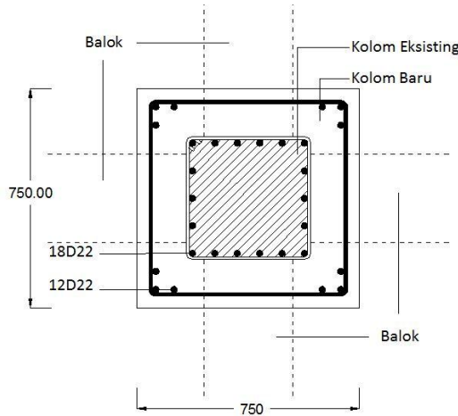
Gambar 4. Penampang Kolom yang Telah Diperbesar
