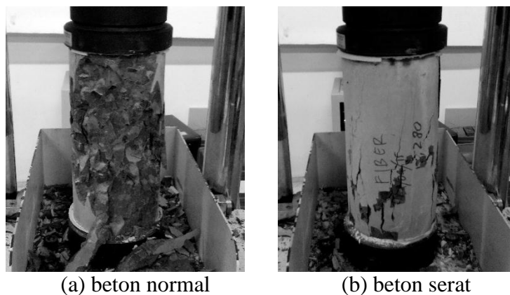
Gambar 5. Hasil Pengujian Kuat Tekan Silinder Beton
