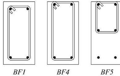
Gambar 2. Konfigurasi Sengkang
