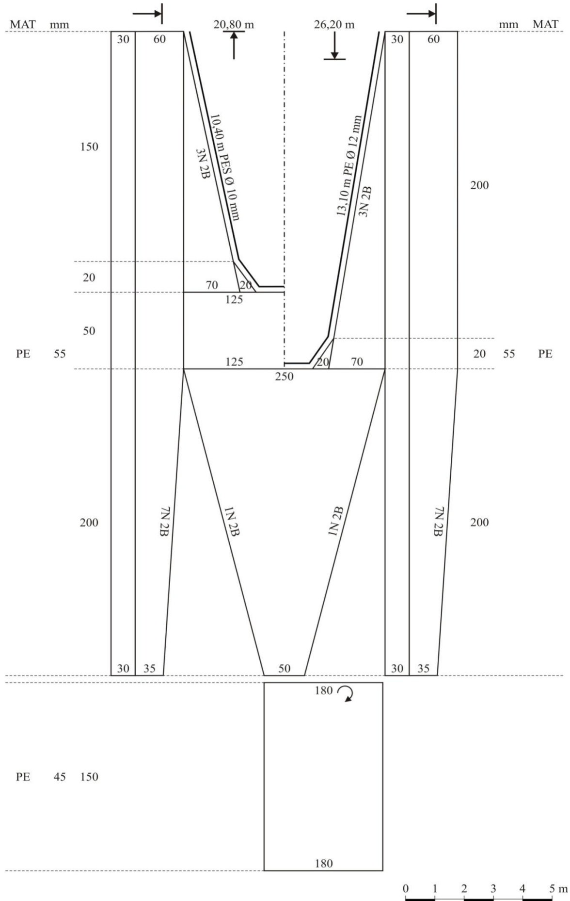
Lampiran 1. Gambar desain pukat udang
