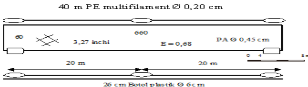
Gambar 2. Konstruksi jaring insang hanging ratio 0,68
