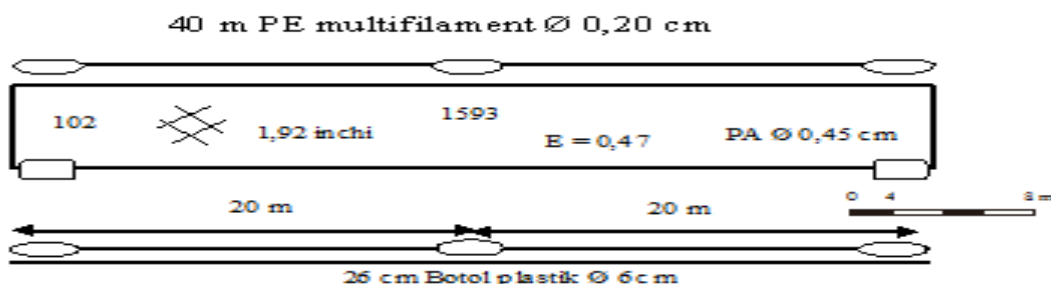
Gambar 1. Konstruksi jaring insang hanging ratio 0,47
