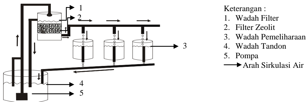
Gambar 1. Desain Resirkulasi
