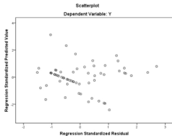
Gambar 4. Uji Heteroskedastisitas
