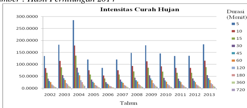
Gambar 4.1. Diagram Intensitas Curah Hujan
