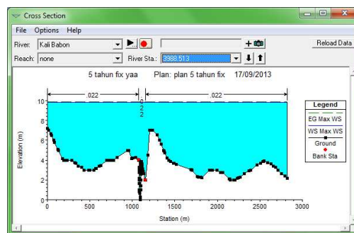
Gambar 3.8 Hasil Plot Muka Air pada Cross Section
