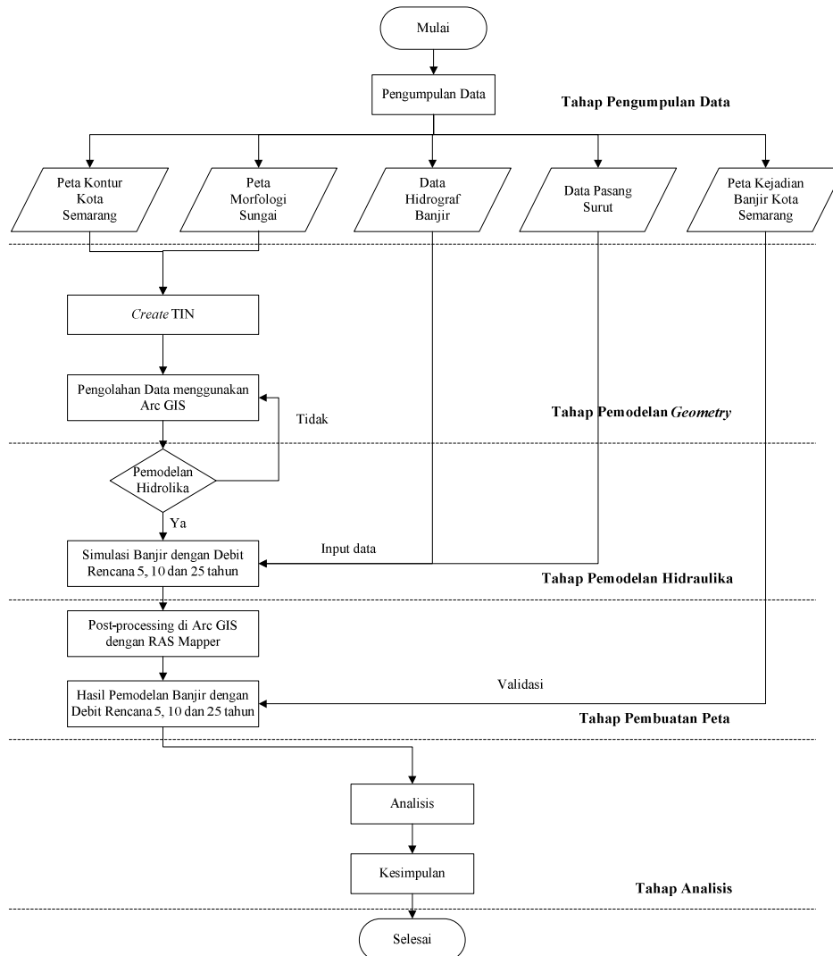
Gambar 3.1 Diagram Alir Metodologi Pelaksanaan Penelitian
