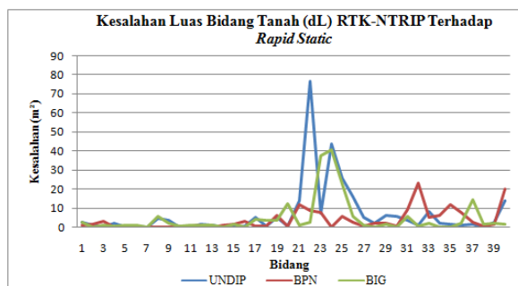
Gambar IV.3. Grafik kesalahan luas bidang tanah (dL) RTK-NTRIP terhadap Rapid Static
