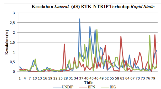
Gambar IV.1. Grafik kesalahan lateral (dS) RTK-NTRIP terhadap Rapid Static
