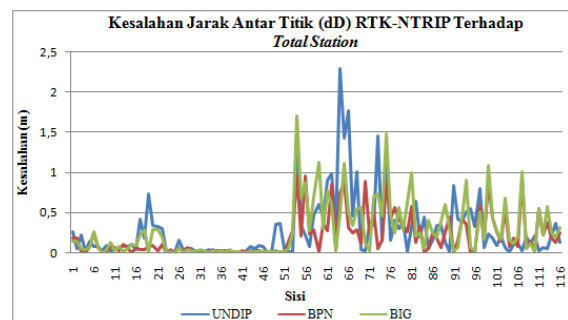
Gambar IV.5. Grafik kesalahan jarak antar titik (dD) RTK-NTRIP terhadap Total Station
