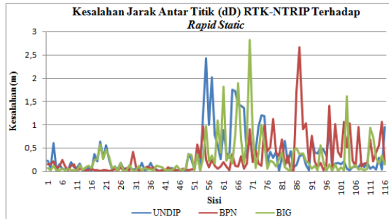
Gambar IV.2. Grafik kesalahan jarak antar titik (dD) RTK-NTRIP terhadap Rapid Static
