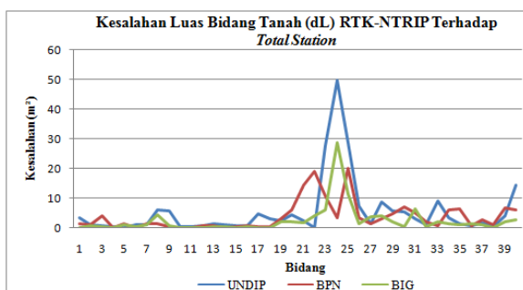
Gambar IV.6. Grafik kesalahan luas bidang tanah (dL) RTK-NTRIP terhadap Total Station
