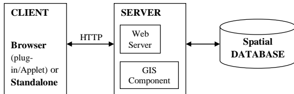
Gambar 2. Arsitektur Sistem Web GIS (Prahasta, 2009)
