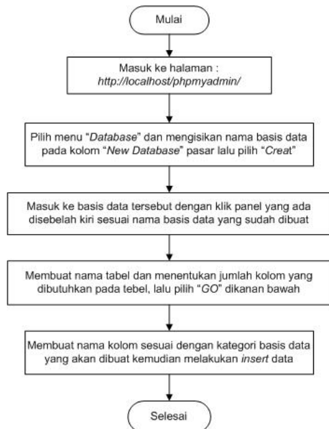
Gambar 6. Diagram Alir Pembuatan Basis Data
