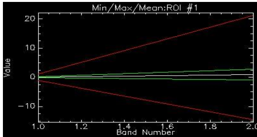
Gambar IV.7 Hasil Korelasi NDVI dengan Suhu Permukaan menggunakan softwre envi 5.0
