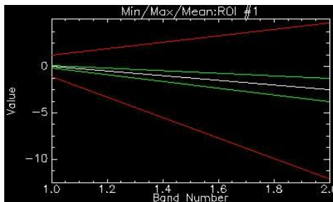
Gambar IV.8 Hasil Korelasi NDVI dengan Suhu Permukaan menggunakan softwre envi 5.0
