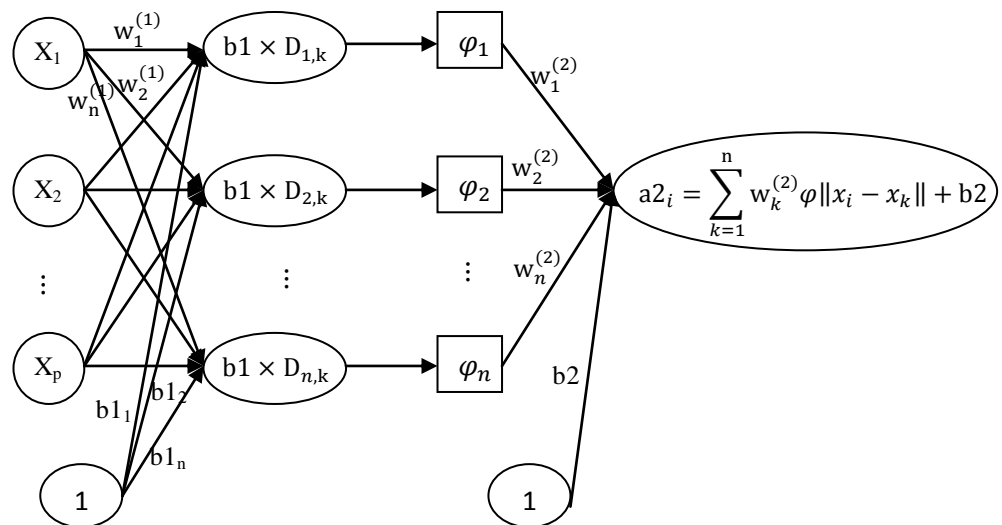
Gambar 1. Arsitektur Radial Basis Function Network
