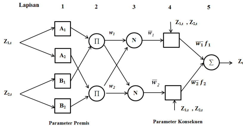
Gambar 1. Arsitektur ANFIS
