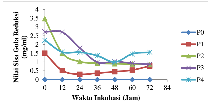
Gambar 2. Sisa gula reduksi S. marcescens pada medium dengan sumber karbon yang berbeda. (P0) = NB (Kontrol); (P1) = NB + 0,5% Glukosa; (P2) = NB + 0,5% Fruktosa; (P3) = NB + 0,5% Maltosa; (P4) = NB + 0,5% Laktosa.
