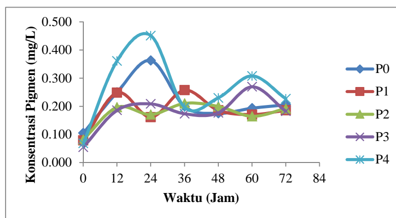
Gambar 4. Produksi pigmen merah S. marcescens pada medium dengan sumber karbon yang berbeda. (P0) = NB (Kontrol); (P1) = NB + 0,5% Glukosa; (P2) = NB + 0,5% Fruktosa; (P3) = NB + 0,5% Maltosa; (P4) = NB + 0,5% Laktosa.
