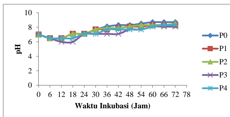
Gambar 3. Derajat keasaman medium pertumbuhan S. marcescens pada sumber karbon yang berbeda. (P0) = NB (Kontrol); (P1) = NB + 0,5% Glukosa; (P2) = NB + 0,5% Fruktosa; (P3) = NB + 0,5% Maltosa; (P4) = NB + 0,5% Laktosa.
